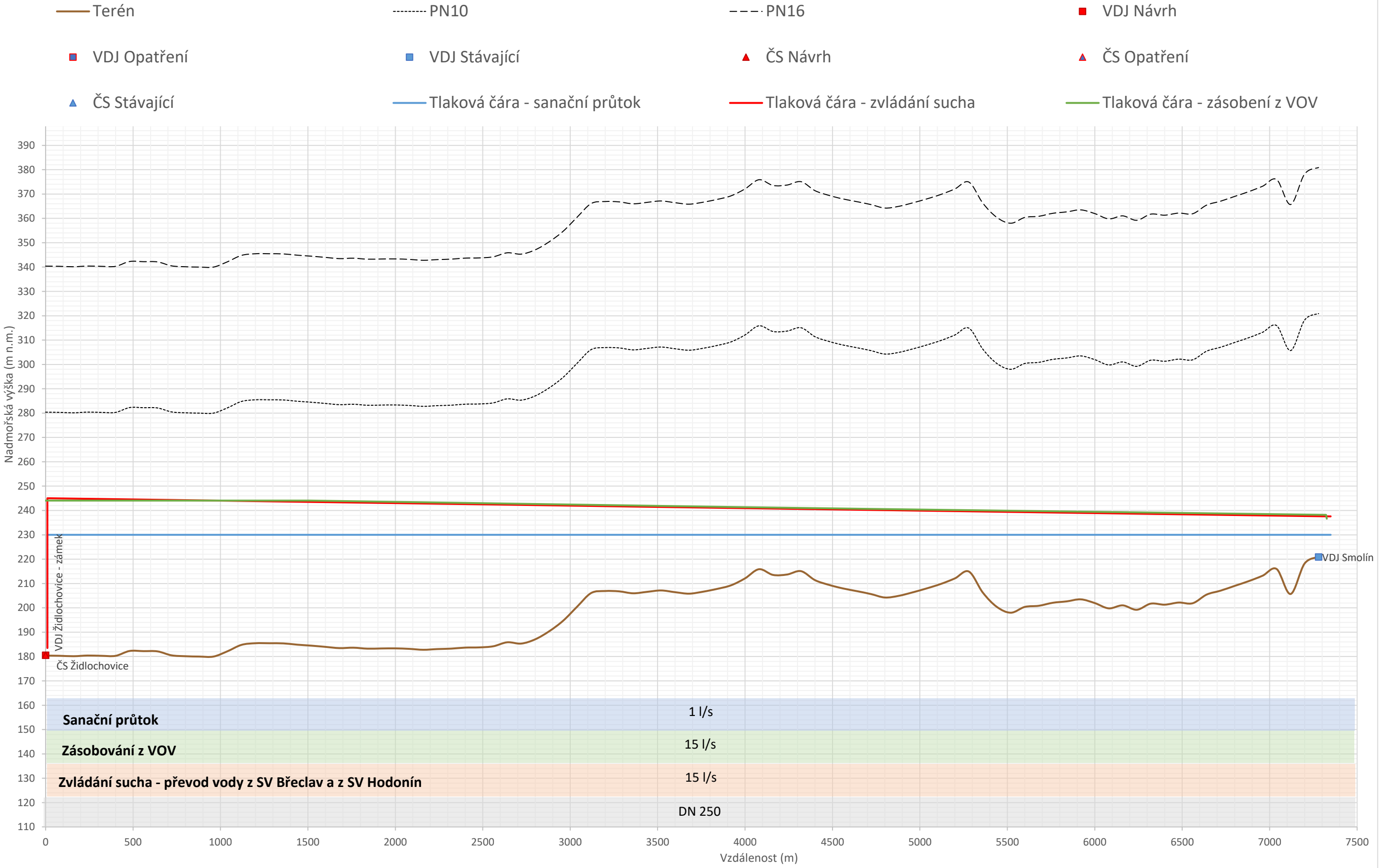
Příloha 9.3: Podrobné podélné profily - Opatření 9. Židlochovice - Pohořelice
