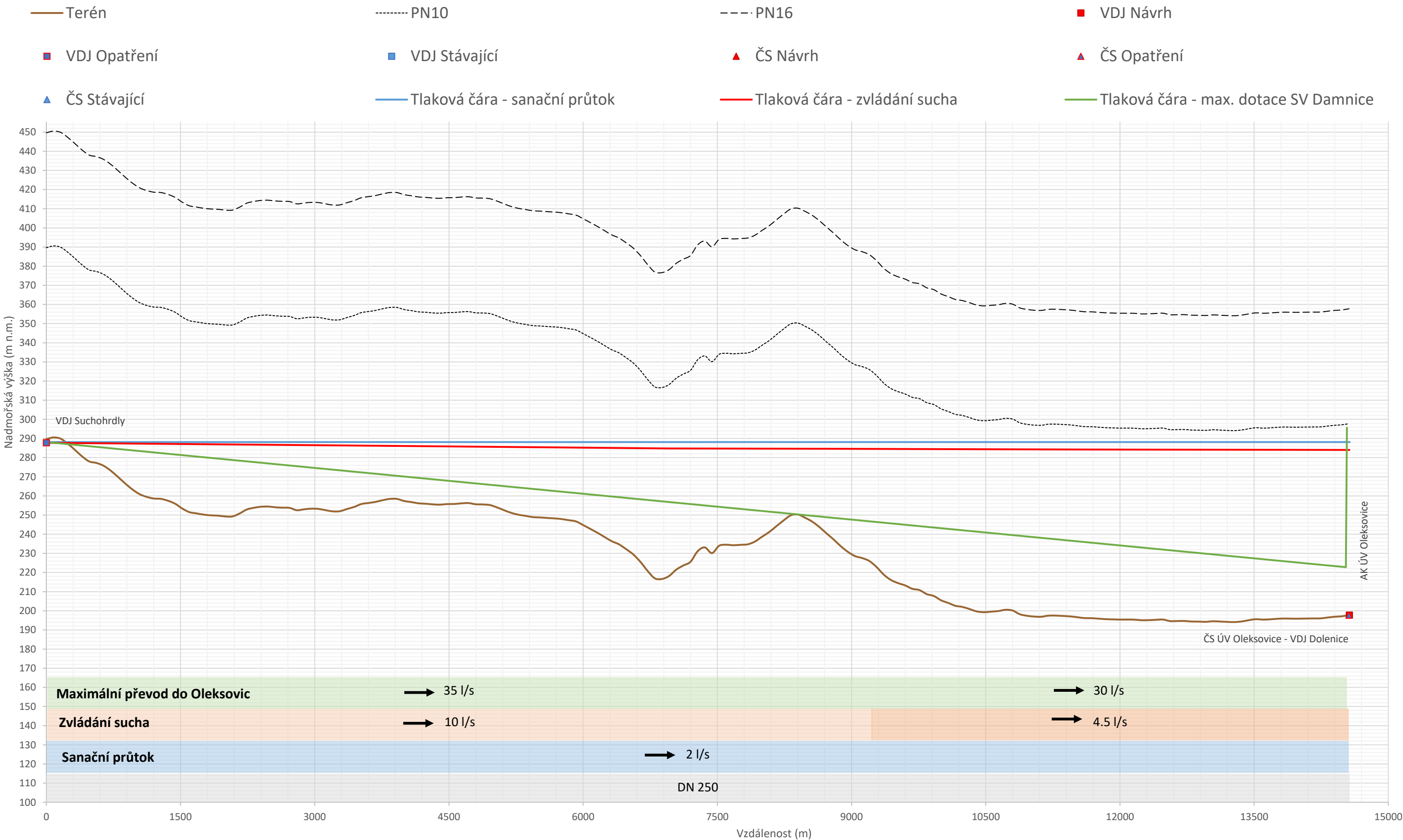
Příloha 7.3: Podrobné podélné profily - Opatření 7. Znojmo - Oleksovice
