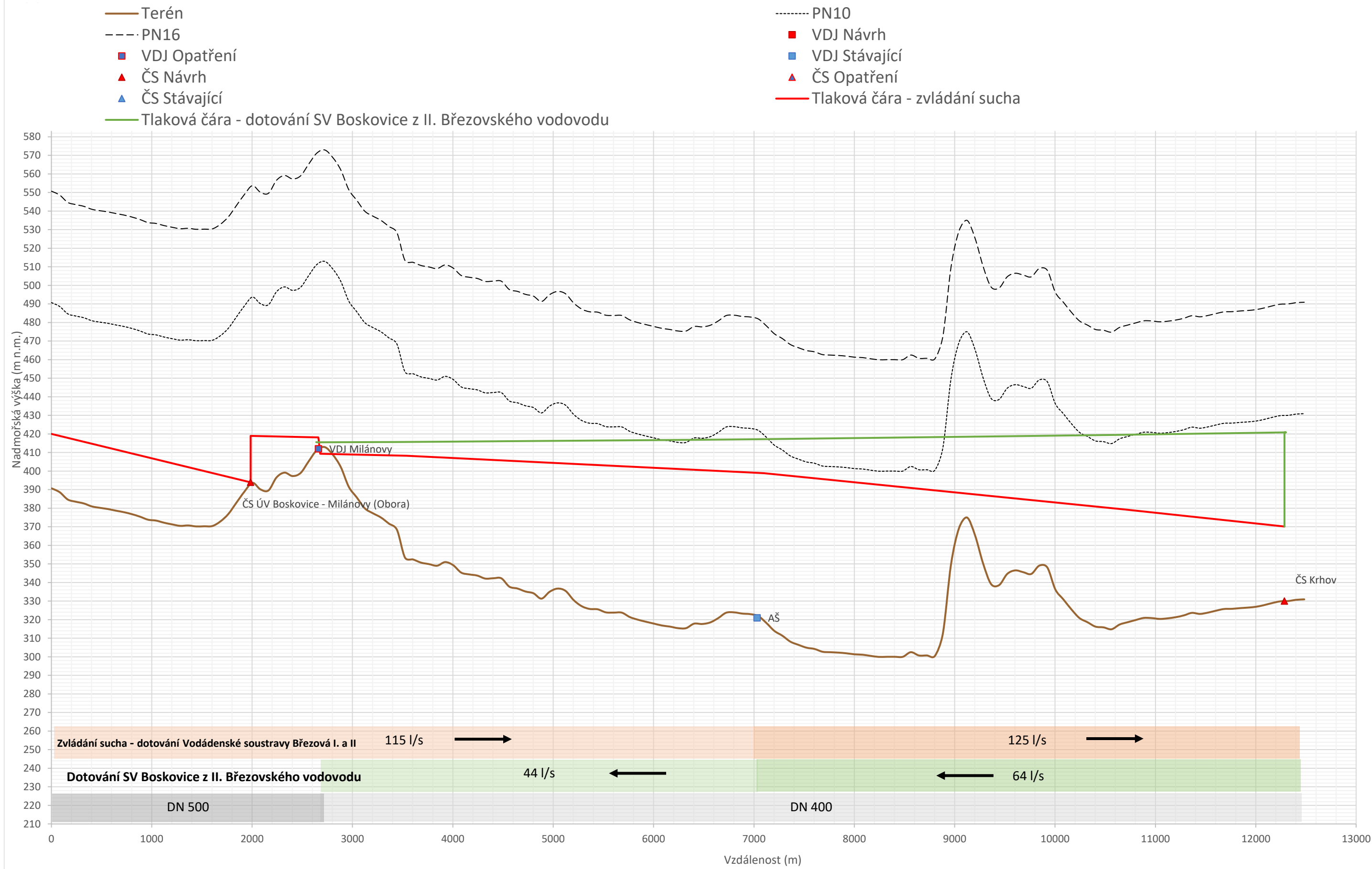
Příloha 5.3: Podrobné podélné profily - Opatření 5. VN Boskovice - Voděrady
