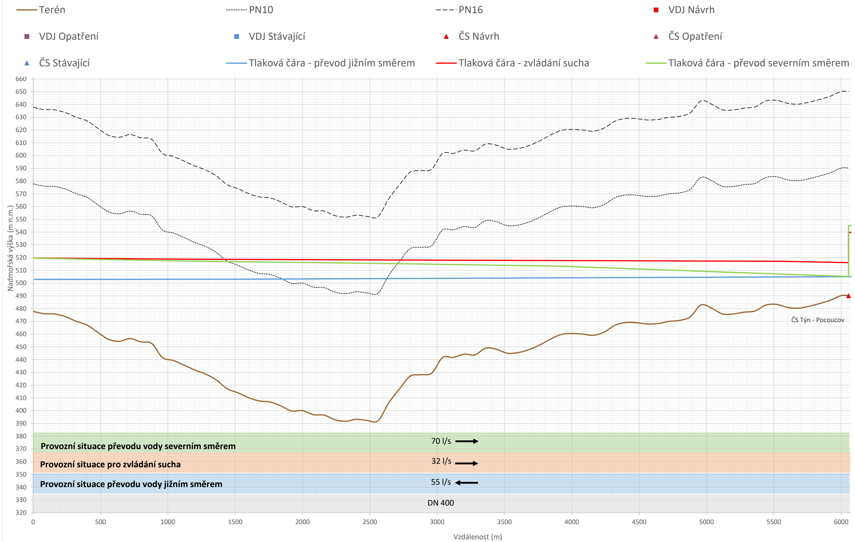
Příloha 28.3: Podrobné podélné profily - Opatření 28. Obchvat Třebíč
