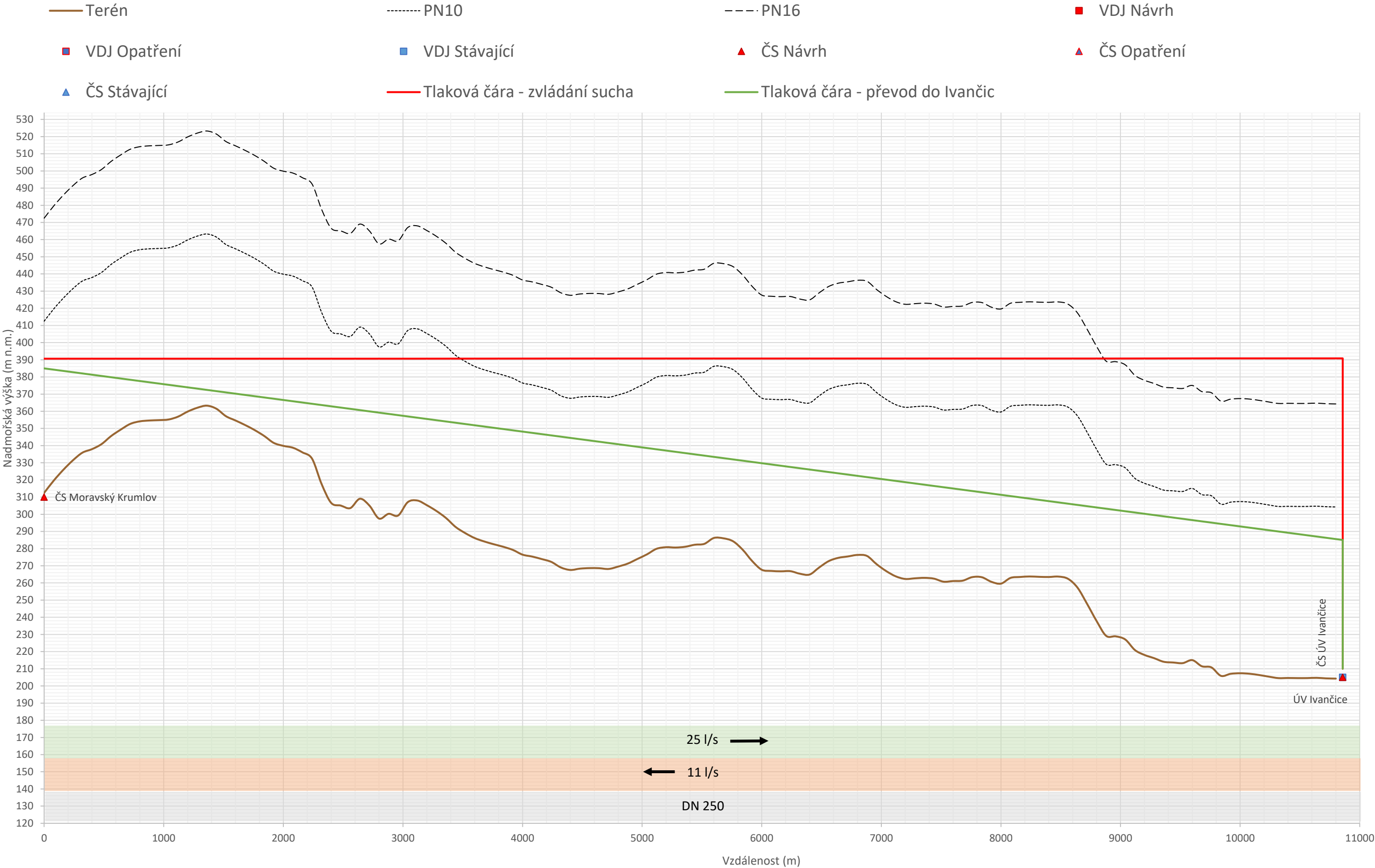
Příloha 26.3: Podrobné podélné profily - Opatření 26. Moravský Krumlov – Ivančice
