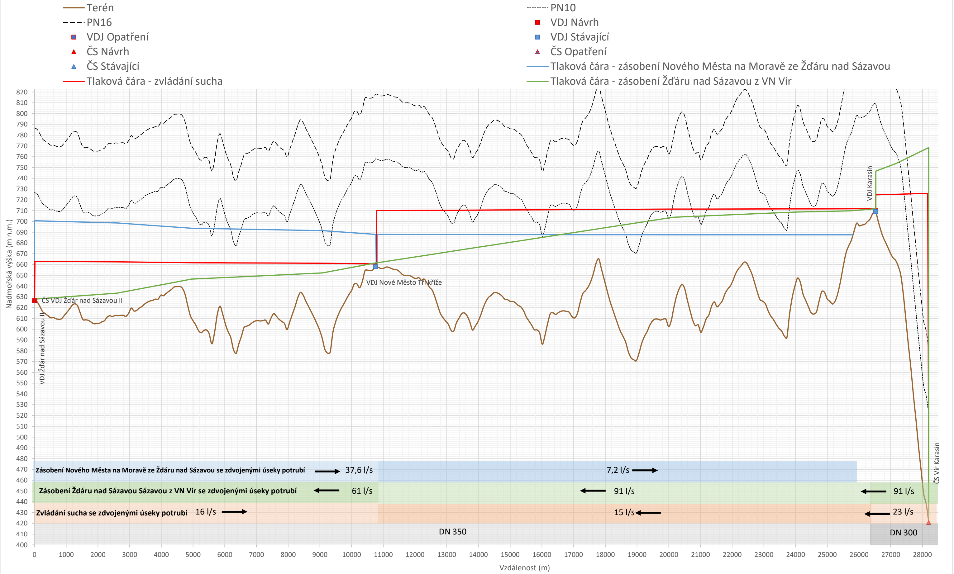
Příloha 21.3: Podrobné podélné profily - Opatření 21. ÚV Vír - Žďár nad Sázavou (úseky se zdvojeným potrubím)
