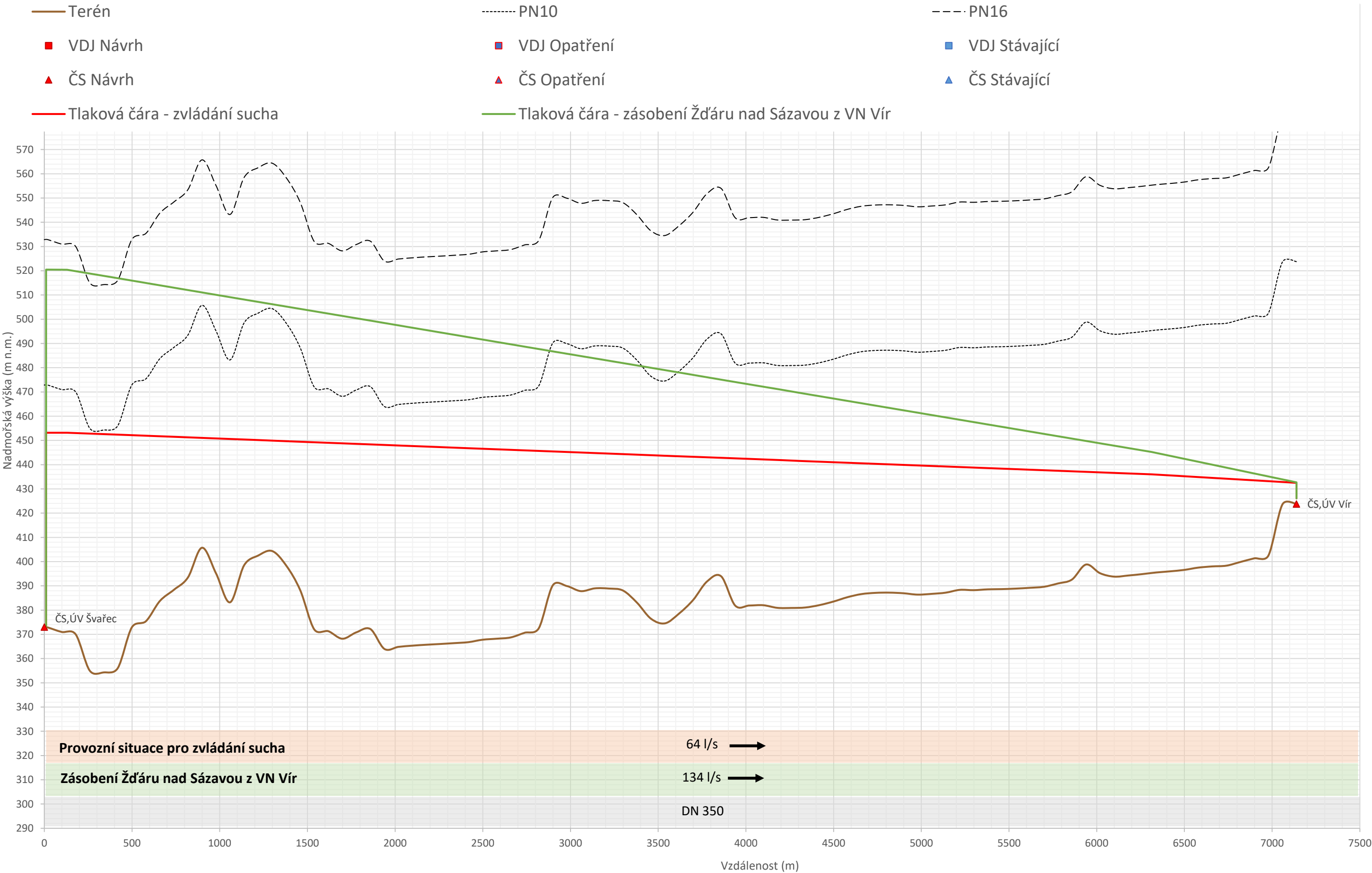
Příloha 20.3: Podrobné podélné profily - Opatření 20. ÚV Švařec - ČS Vír
