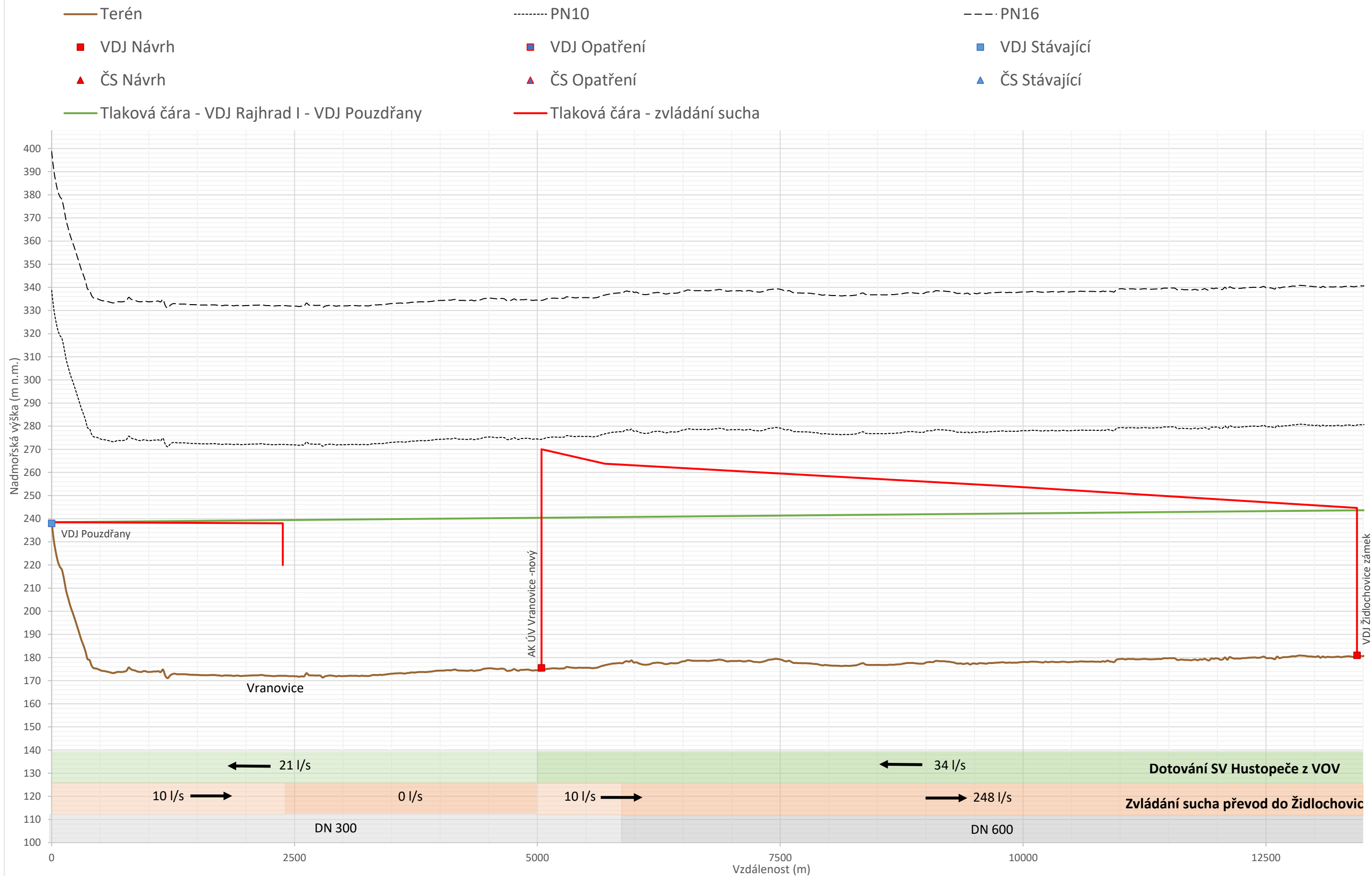
Příloha 2.3: Podrobné podélné profily - Opatření 2. Hustopeče - Vranovice - Židlochovice
