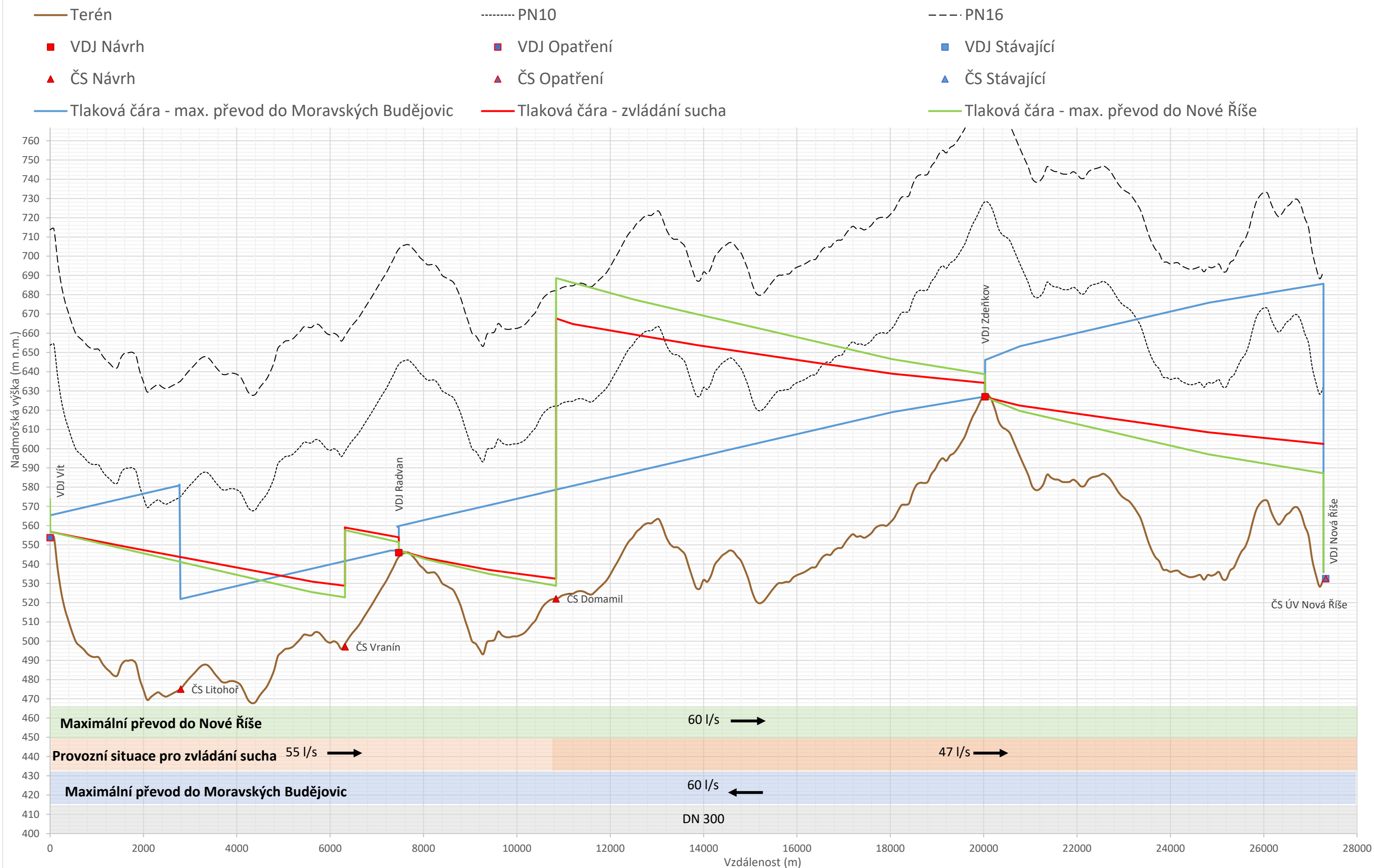
Příloha 17.3: Podrobné podélné profily - Opatření 17. Moravské Budějovice - Nová Říše
