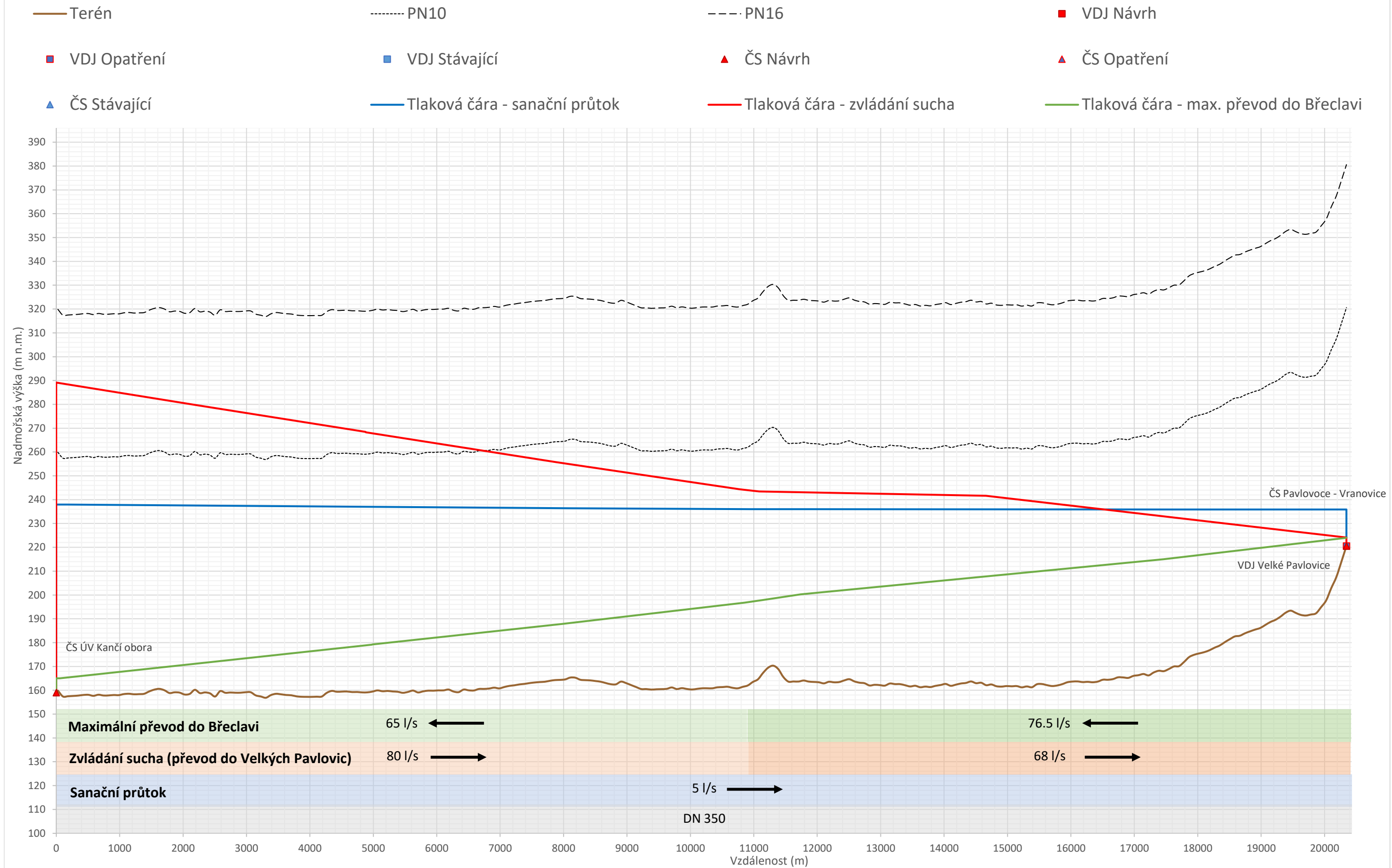
Příloha 1.3: Podrobné podélné profily - Opatření 1. Břeclav - Podivín - Velké Pavlovice
